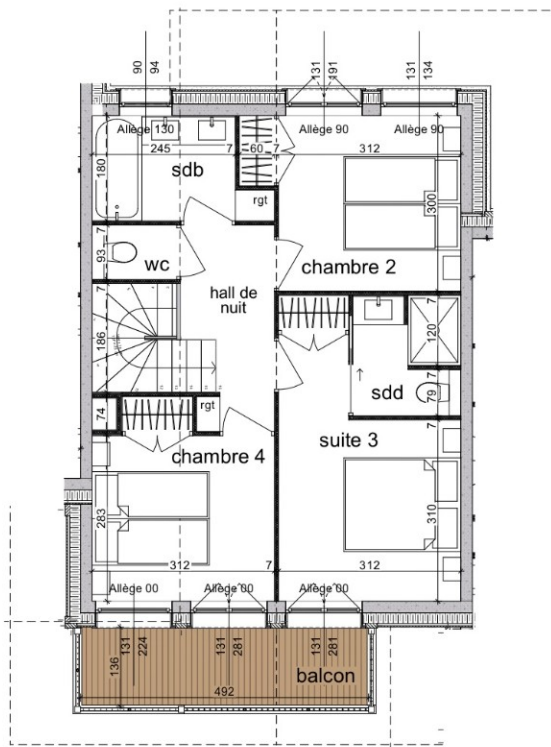
Etage 2
